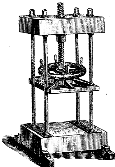
Рис. 36-й. Паковальный пресс большой величины, также же- лѣзный, но съ деревянн. нижн. и верхн. досками.
