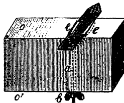
Рис. 90-й. Правая колодка гобели, повернутая низомъ ( o ) вверхъ, а верхомъ ( o' ) внизъ; n —рѣзакъ; a —проходящій внутри колодки болтикъ, обозначенный точечн. линіями; e и e —лапки болтика; o —гайка, навинчиваемая на верхній конецъ болтика.
