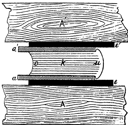
Рис. 110-й. Зажиманіе книги для волоченія головки или хвоста. Буквы имѣютъ то-же значеніе, что на рис. 109-мъ.
