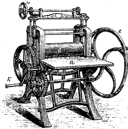
Рис. 40-й. Сатинировавшая машина.
