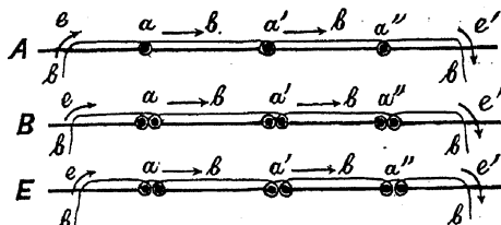
Рис. 78-й. Веденіе нитки при шиваніи на шнурахъ безъ пропилки корешка—швомъ итолкою назадъ . А—шиваніе на оди- ночныхъ шнурахъ; В и Е—шиваніе на двойныхъ шнурахъ.
